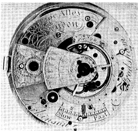
Figura 3 Movimento di orologio da tasca firmato Parkinson & Frodsham. Presenta la rara applicazione di una speciale forma di compensazione termica della spirale del bilanciere, simile al "sugar tong" di Earnshaw. (vedi riquadro a pag.4).
